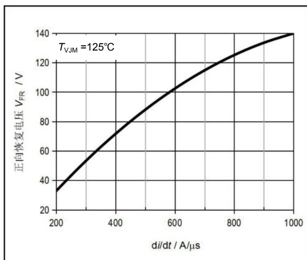
图7. 正向恢复电压与开通 di/dt 的关系曲线
